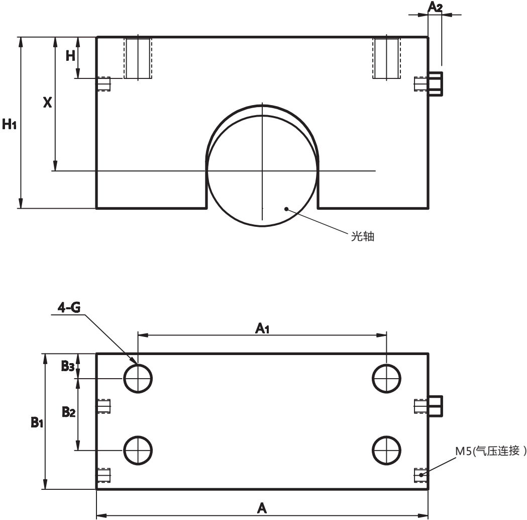
尺寸图
