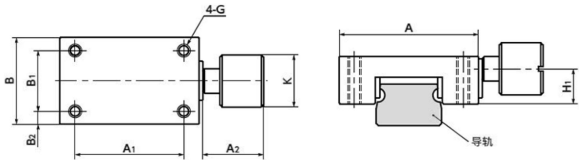
尺寸图
