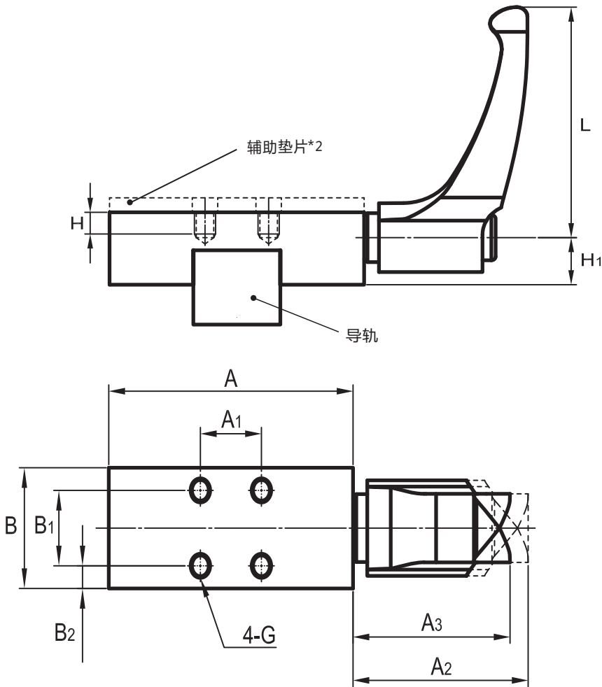
尺寸图
